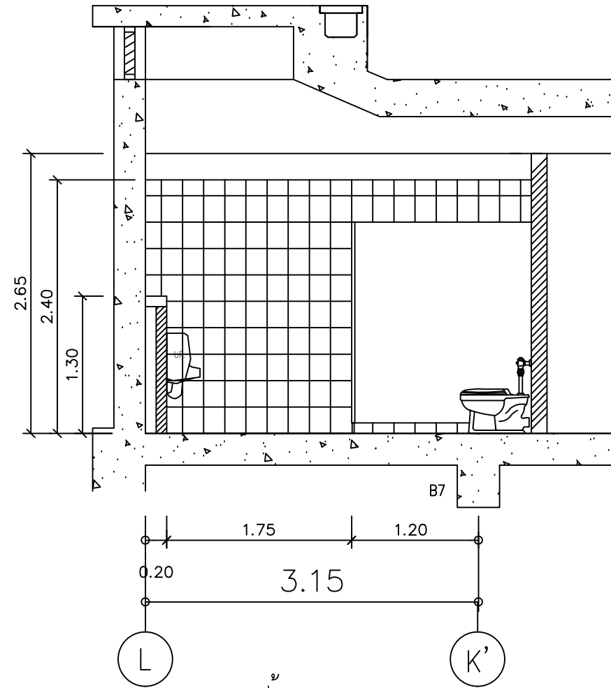
รูปด้าน 8 SCALE 1 : 50
