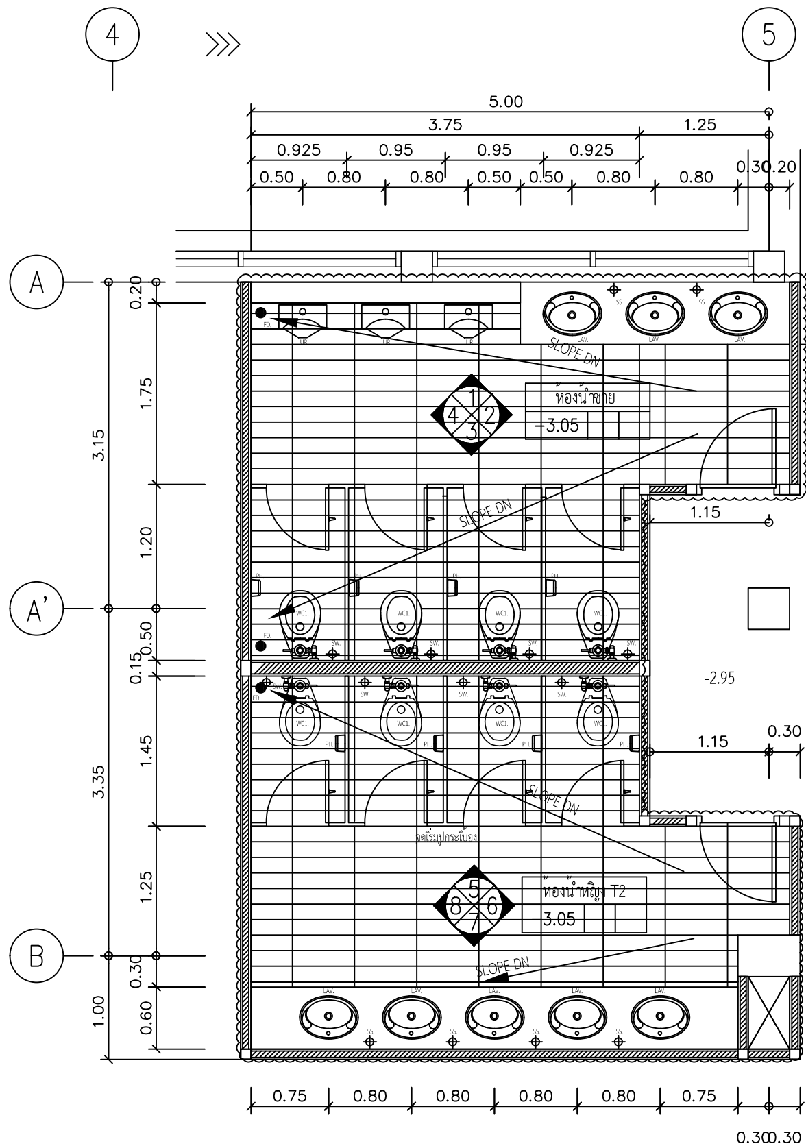
แปลนรื้อถอนห้องน้ำชาย-หญิง (ฝั่งอาคารวิจัยและการศึกษาต่อเนื่อง) SCALE 1 : 50
