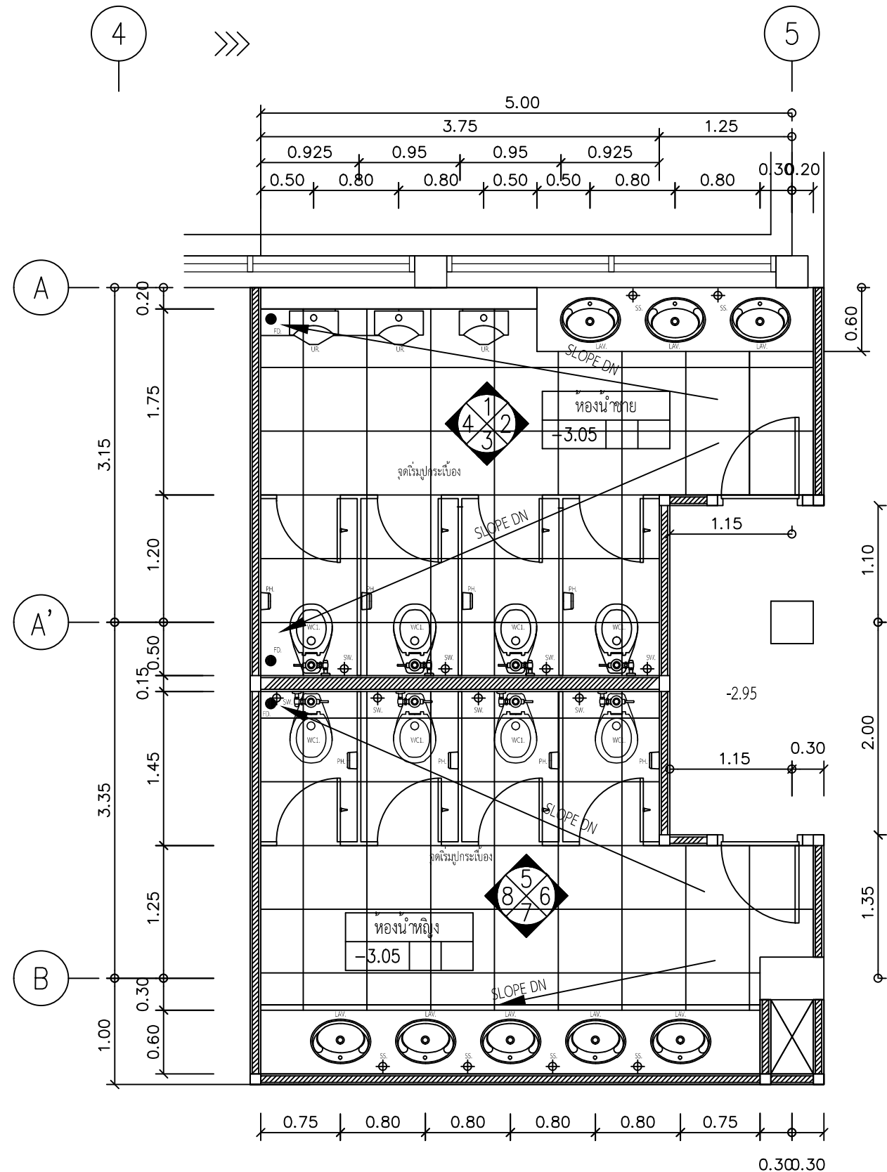
แปลนปรับปรุงห้องน้ำชาย-หญิง ฝั่งอาคารวิจัยและการศึกษาต่อเนื่อง
