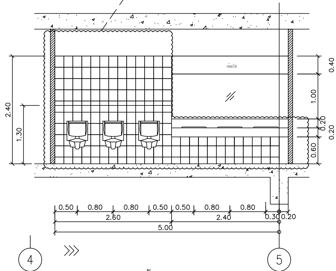
รูปดำน 1 SCALE 1 : 50
