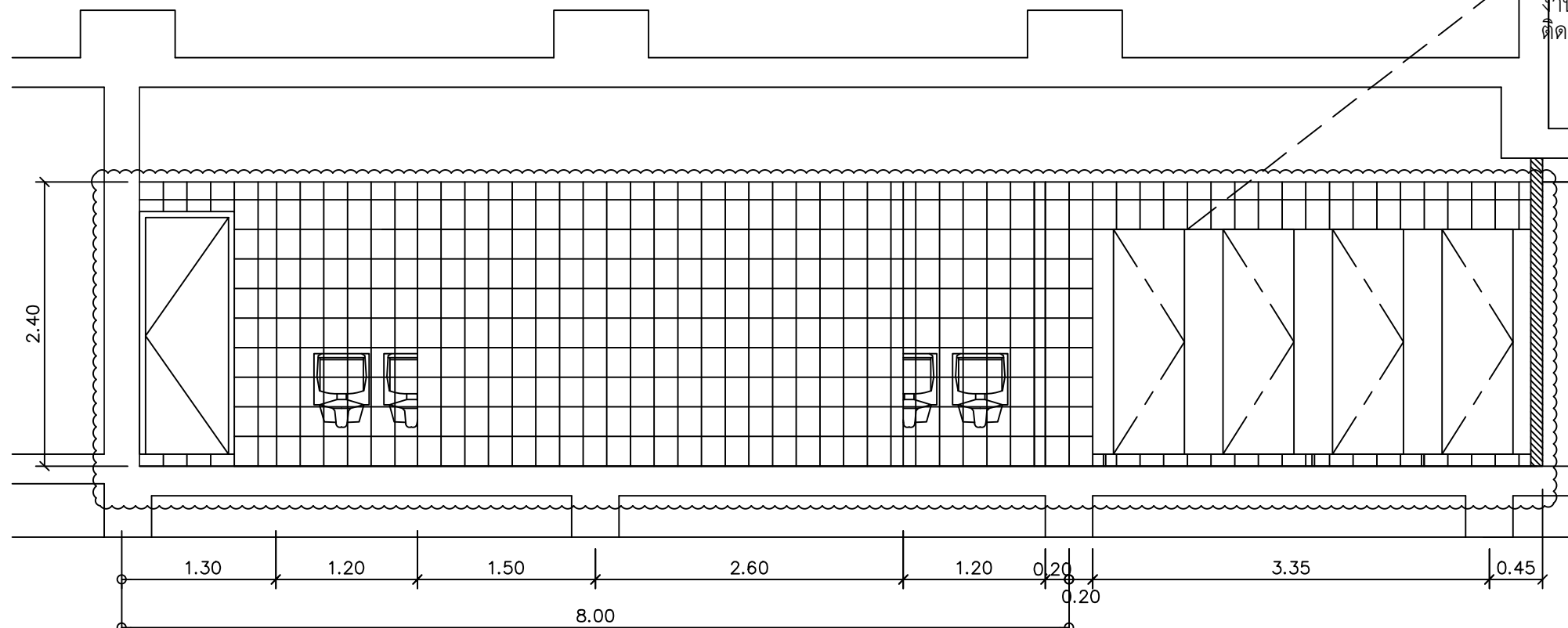
รูปดำน 3 SCALE 1 : 50
