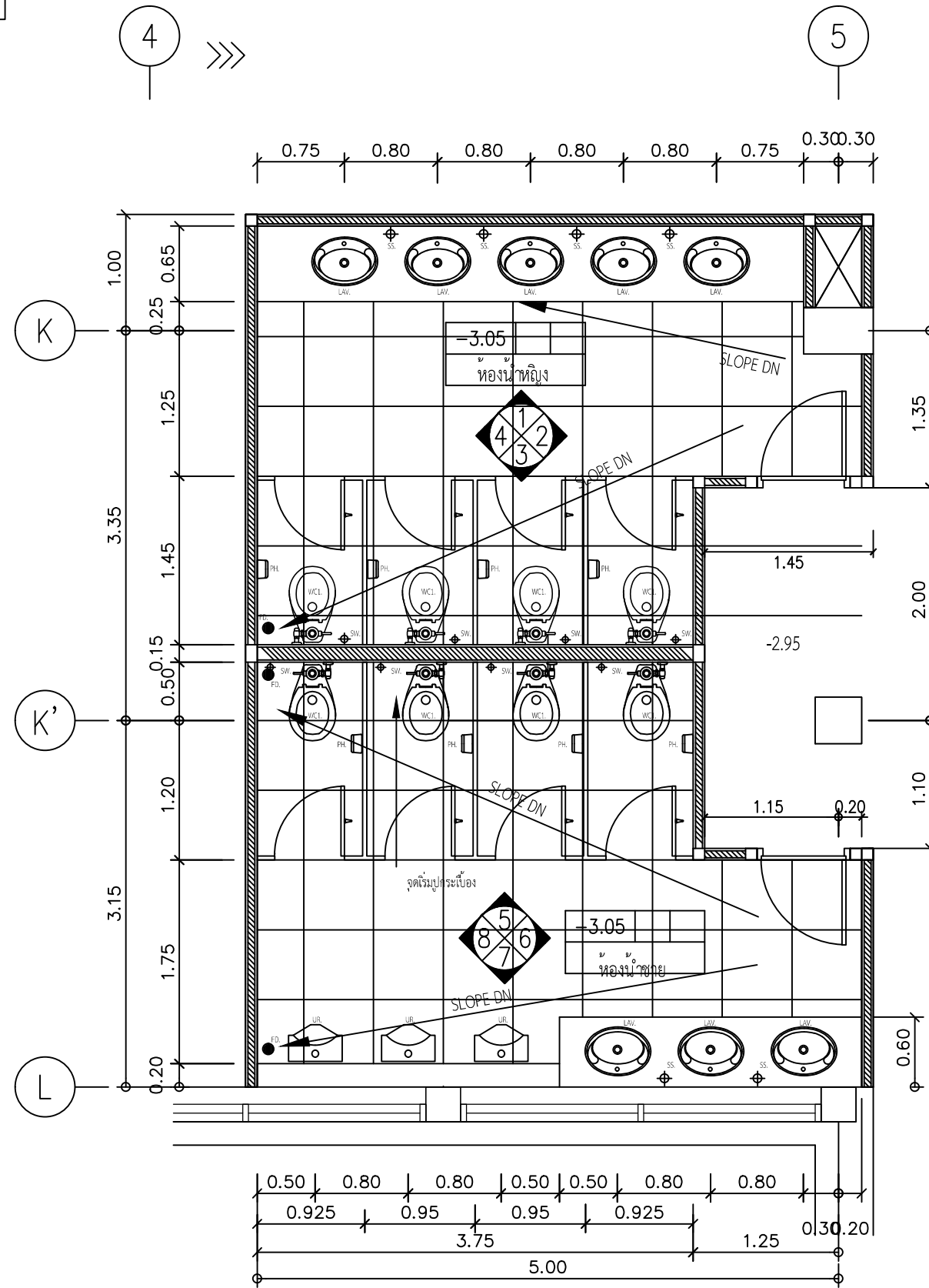
แปลนปรับปรุงห้องน้ำหญิง-ชาย (ฝั่งอาคารคณะศึกษาศาสตร์)
