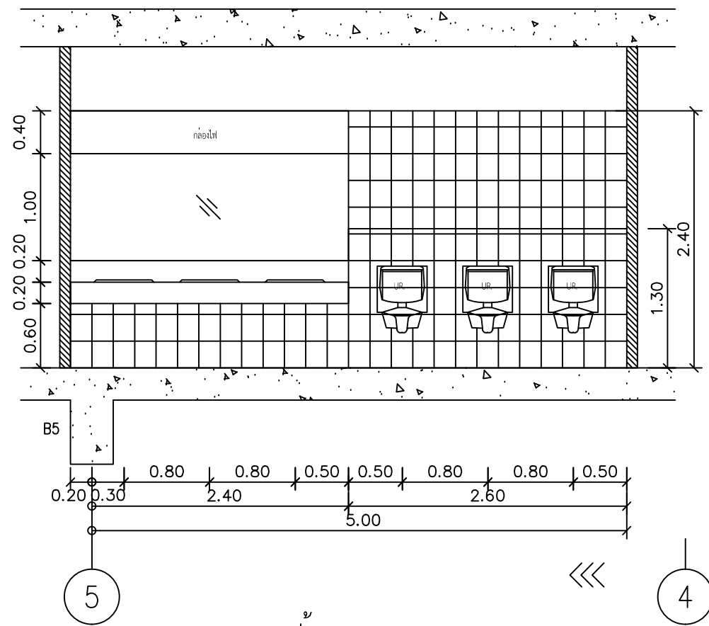
รูปด้าน 7 SCALE 1 : 50
