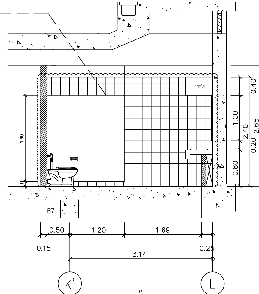
รูปดำน 2 SCALE 1 : 50
