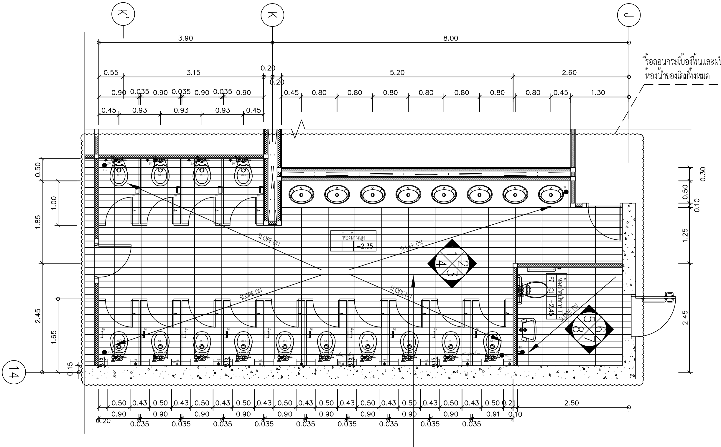
แปลนรื้อถอนห้องน้ำหญิงและคนพิการ (ฝั่งอาคารคณะสังคมศาสตร์)
