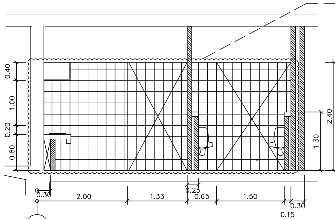
รูปด้าน 2 SCALE 1 : 50
