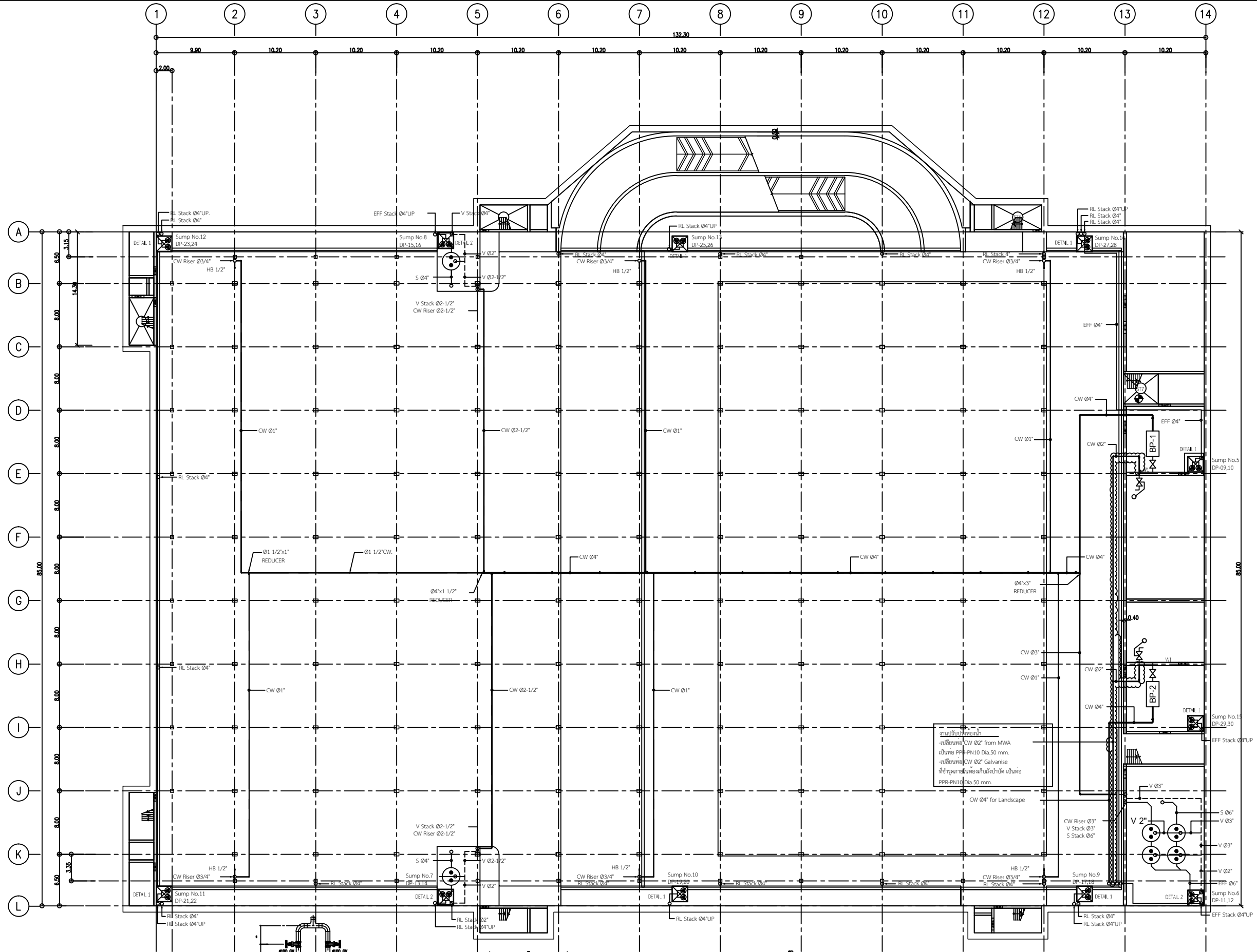
แปลนระบบสุขาภิบาลชั้นใต้ดิน 2 (B2) Scale 1:500
