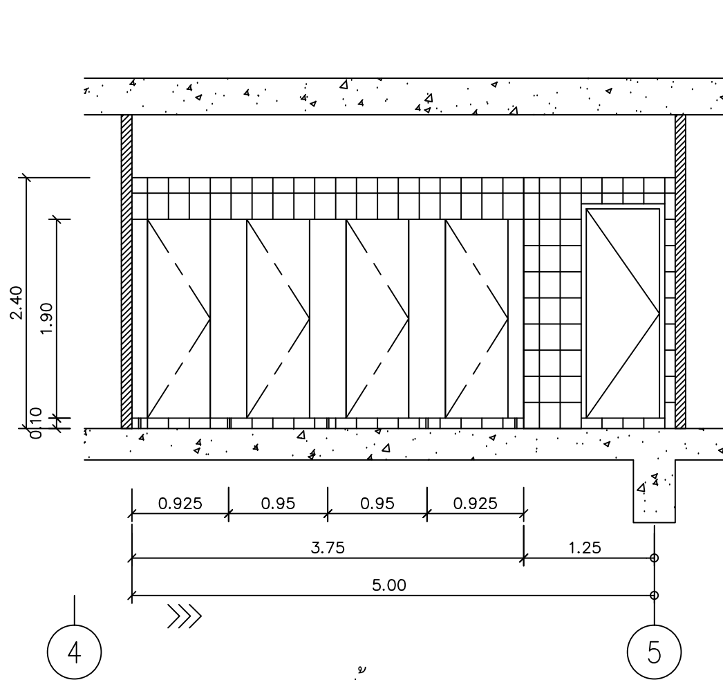
รูปด้าน 5 SCALE 1 : 50
