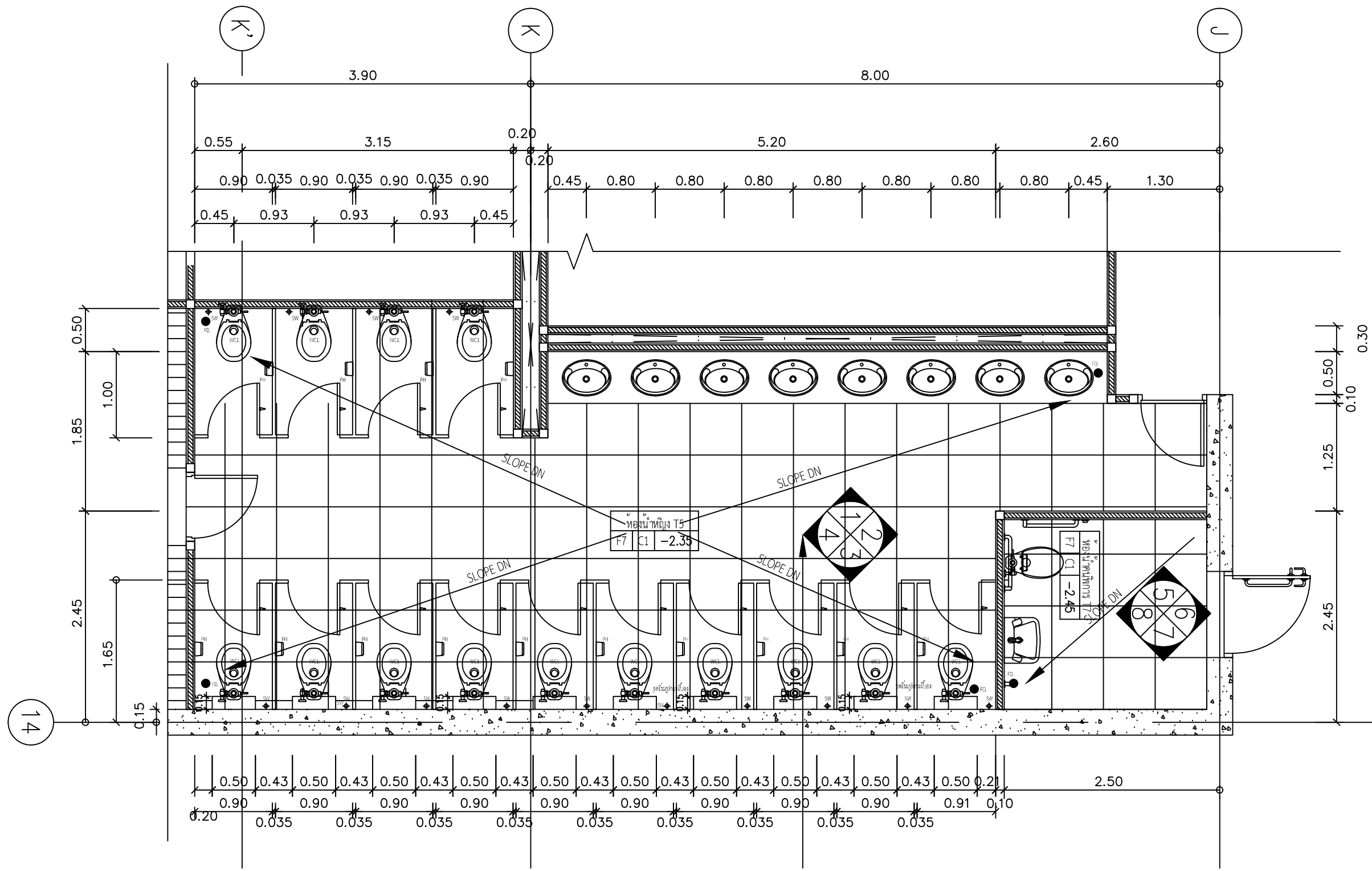
แปลนปรับปรุงห้องน้ำหญิงและคนพิการ (ฝั่งอาคารคณะสังคมศาสตร์)
