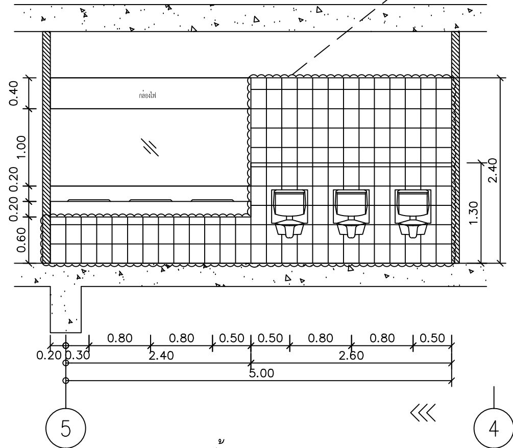
รูปดำน 3 SCALE 1 : 50
