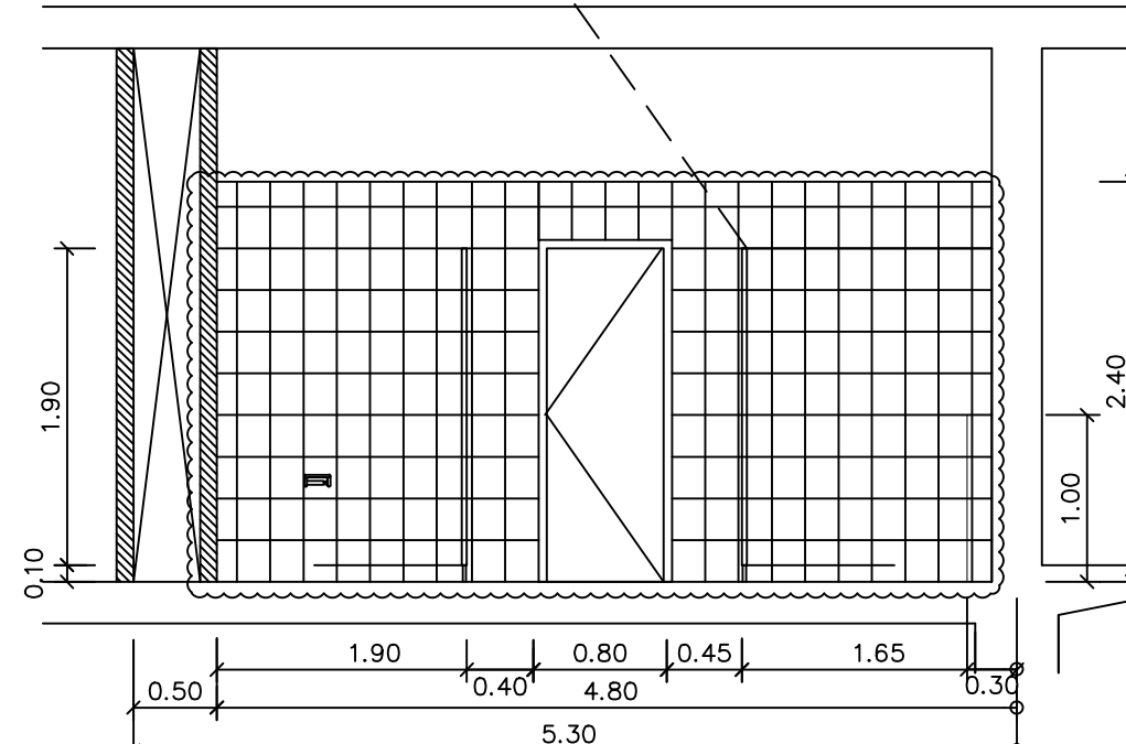
รูปด้าน 4 SCALE 1 : 50
