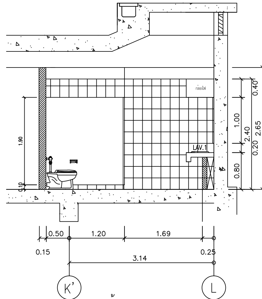
รูปด้าน 6 SCALE 1 : 50
