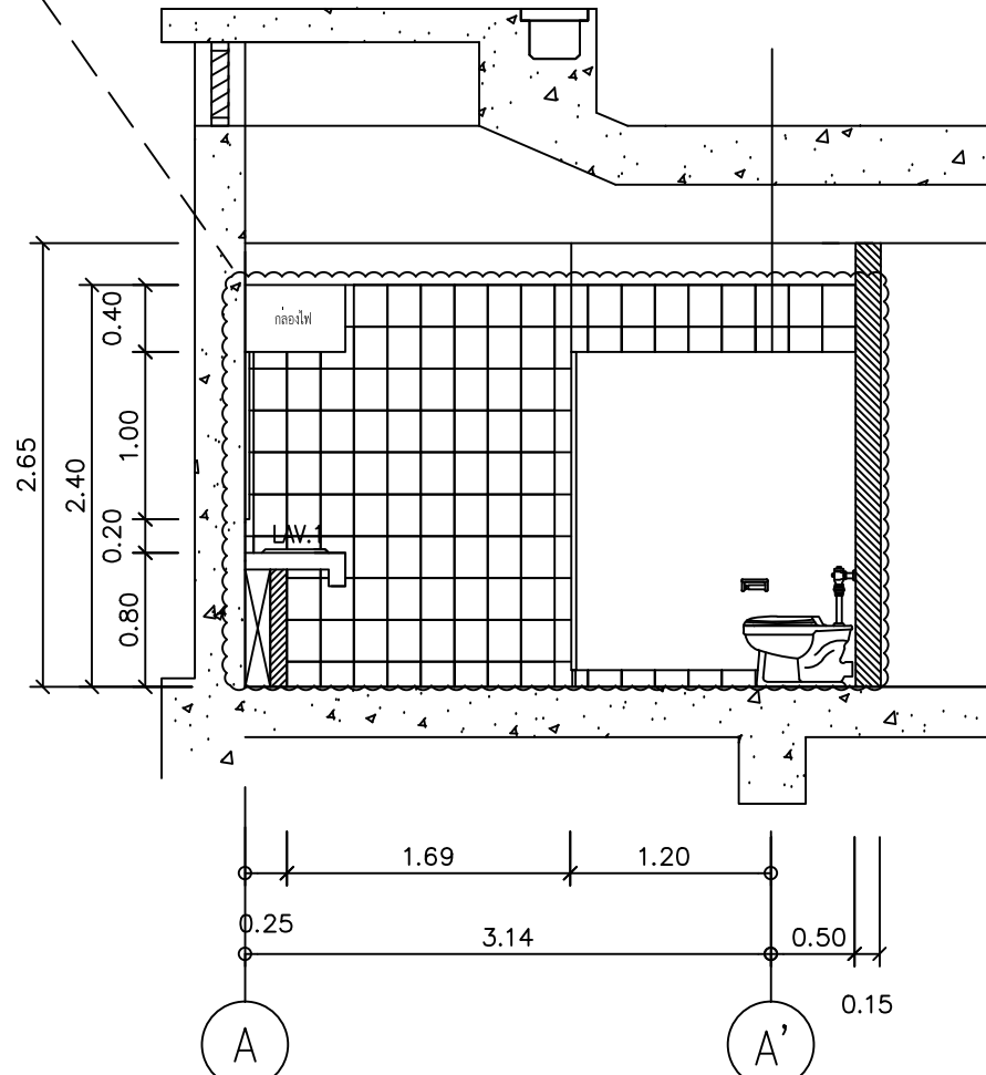
รูปดำน 2 SCALE 1 : 50
