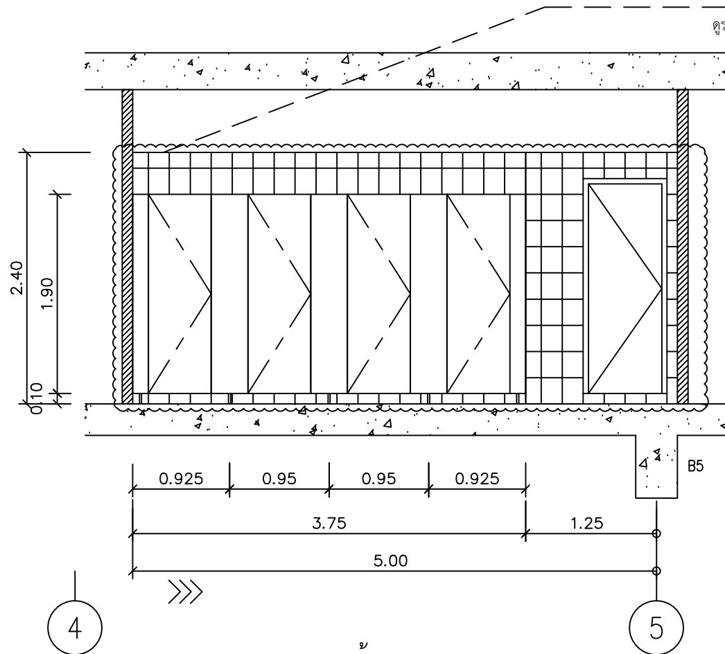
รูปดำน 1 SCALE 1 : 50
