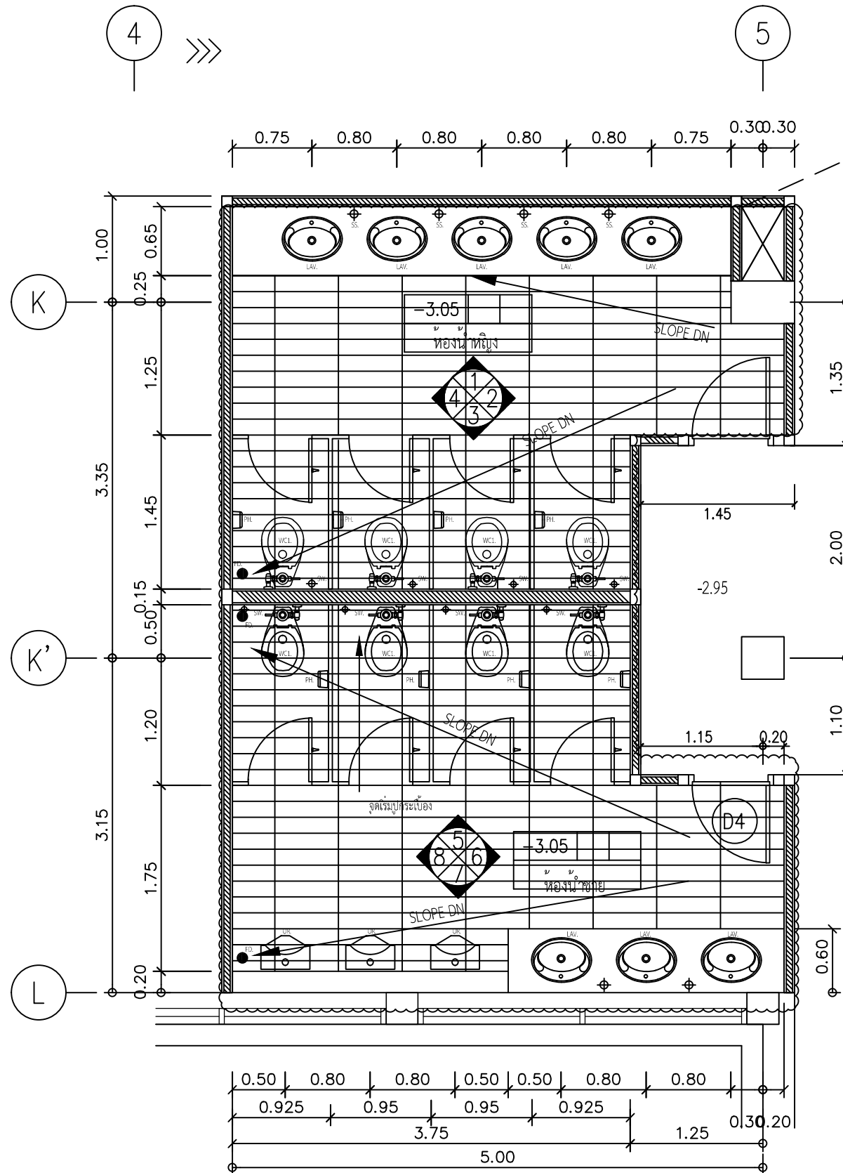
แปลนรื้อถอนห้องน้ำหญิง-ชาย (ฝั่งอาคารคณะศึกษาศาสตร์)
