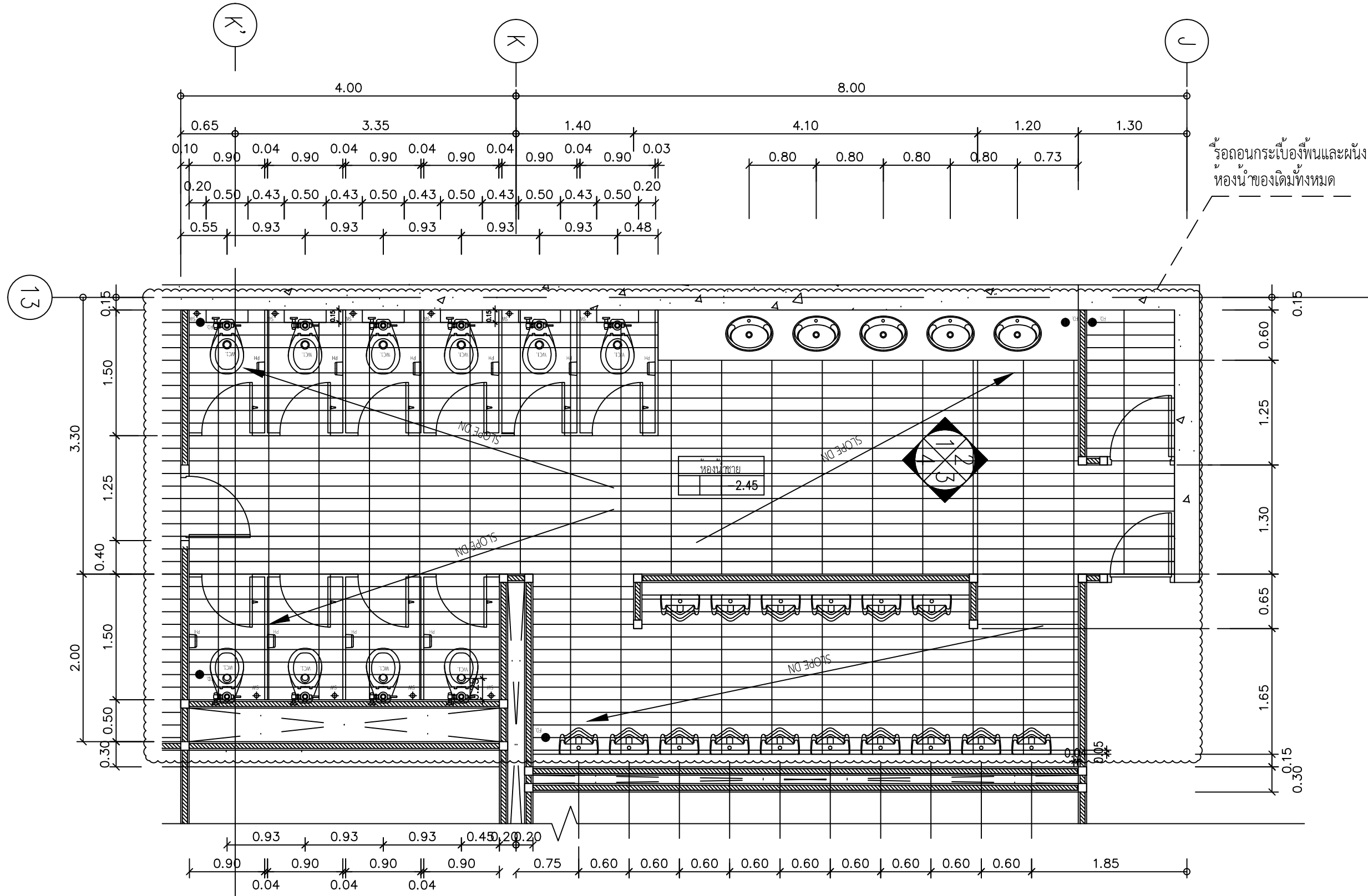
แปลนรื้อถอนห้องน้ำชาย (ฝั่งอาคารคณะสังคมศาสตร์)
